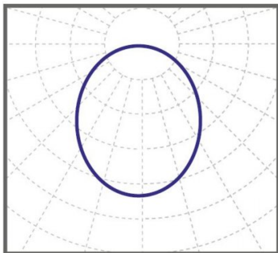
косинусная Д КСС 95°
