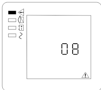
Рисунок 10 – Пример отображения кода неисправности на ЖК-дисплее.
