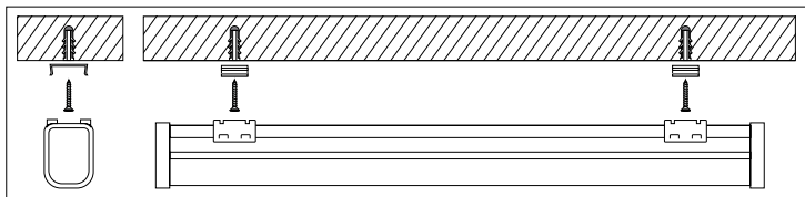
Рис. 2. Схема установки светильника
