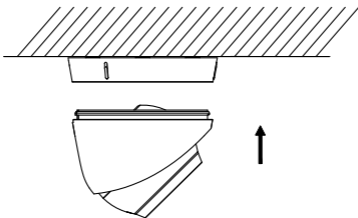
Рисунок 2-4-4 Установка камеры на платформу
