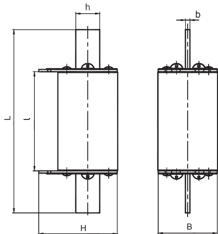
Размеры для справок. Рисунок Б.2. Плавкая вставка
