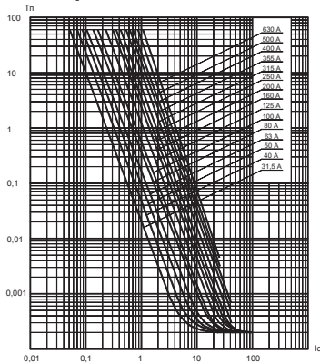
Рисунок В.1. Предохранители ПН2-100, ПН2-250, ПН2-400, ПН2-600
