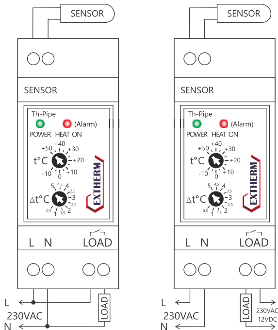
Схема подключения
