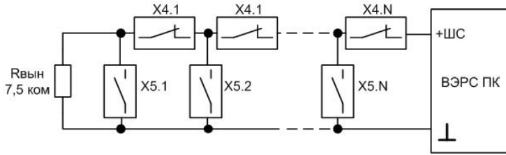
Рисунок Б10. Схема включения охранных извещателей в ЩО.
